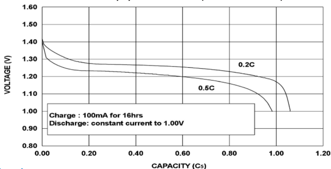
Charakterystyka rozładowania (load 0.2C - 200 mA):
