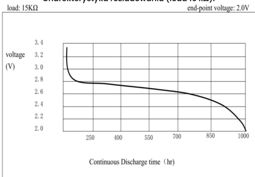
Charakterystyka rozładowania (load 15 kΩ):
