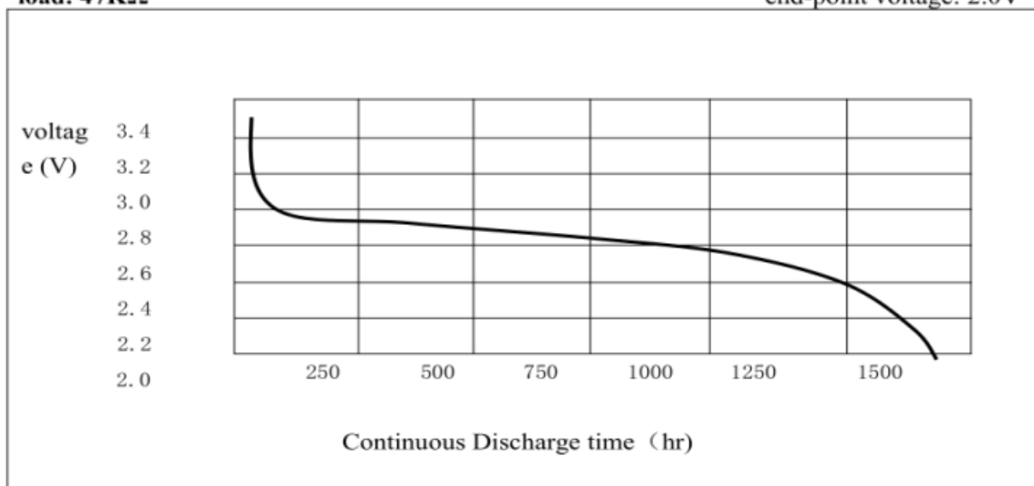
load: 47KΩ Charekterystyka rozładowania (load 47 kΩ): end-point voltage: 2.0V
