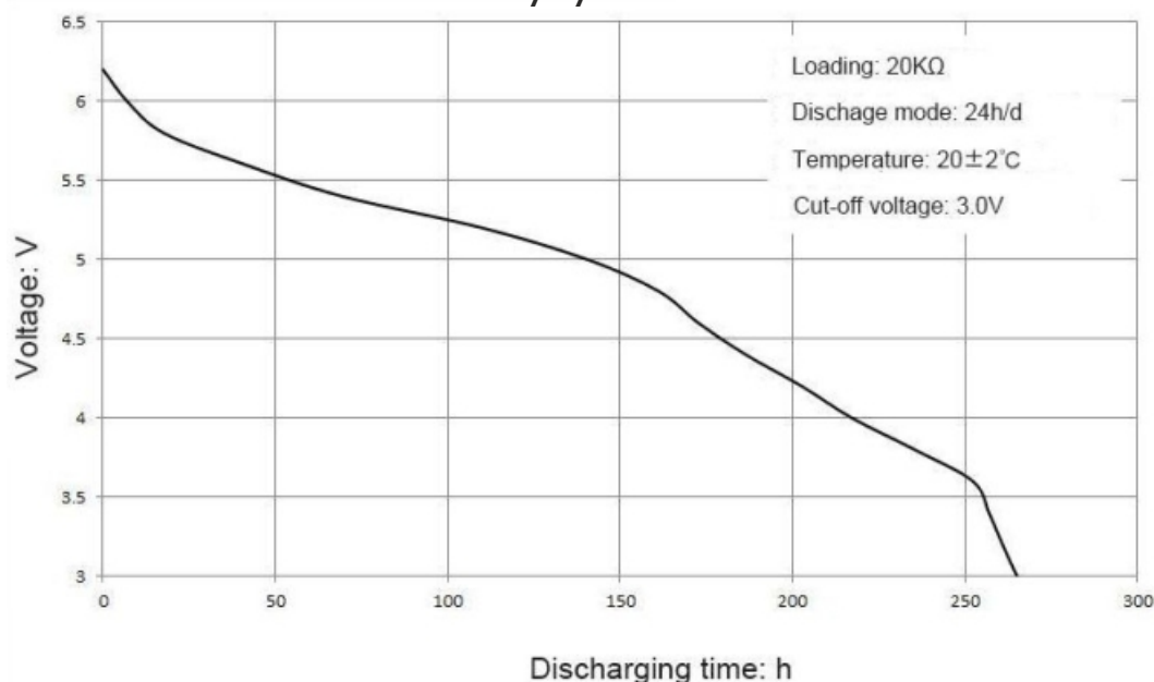
Charekterystyka rozładowania:
